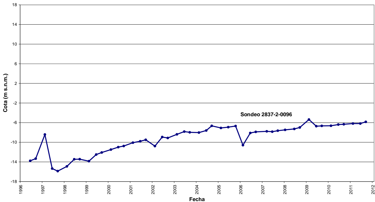
Figura 7. Evolución piezométrica, años 1996-2012. Piezómetro 2837-2-0096, ubicado en figura 8.
