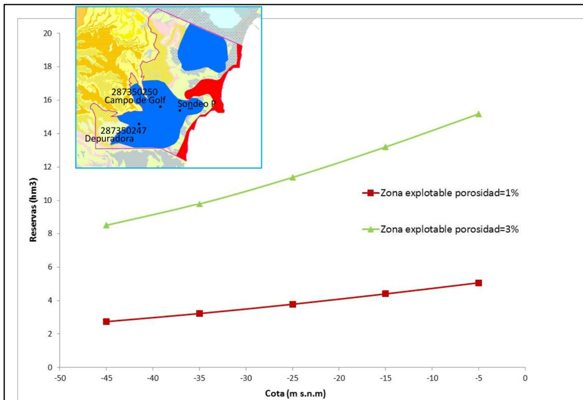
Figura 24. Curvas de explotación del acuífero Cabo Roig desde un posible sondeo situado al este de Campo de Golf (coordenadas del sondeo X=697250; Y=4198800).
