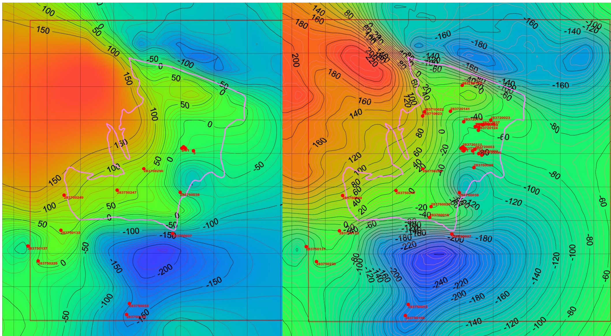
Figura 15. Mapa isobatas del Techo (izquierda) y Muro del acuífero Plioceno de Cabo Roig (perímetro en rosa). En rojo: límites del modelo 3D (retícula cada 2 km).
