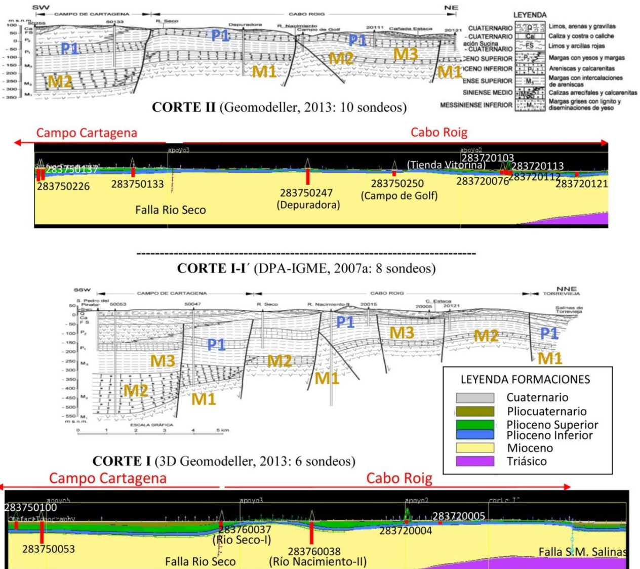
Figura 5. A color: cortes hidrogeológicos I y II del área de Cabo Roig computados por 3D Geomodeller; blanco y negro, mismos cortes según informe DPA-IGME, 2007 a .
