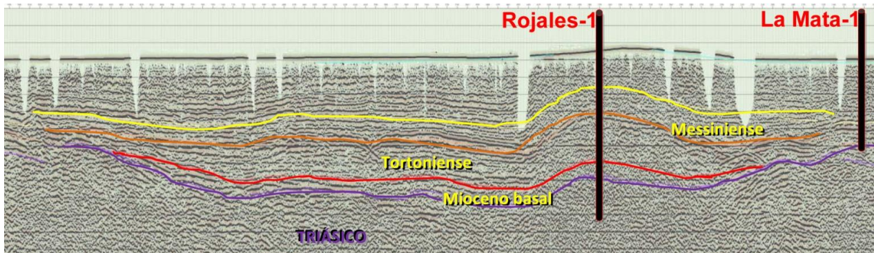
Figuras 21. Línea S-84-68. (22 km) Se observa estructura antiformal en las proximidades de Rojales -1. La Mata-1 corta Triás a 759m (Log final, Ministerio Industria 1970, Servicio Hidrocarburos, 1153).
