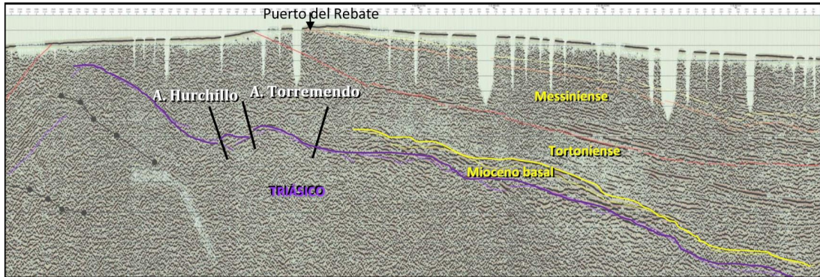
Figura 19. Línea 84-64(34.8 km), caracterizando la geometría de la Cuenca del Campo de Cartagena, justo al sur de Cabo Roig, entre la línea de costa y el antiforme de Torremendo.
