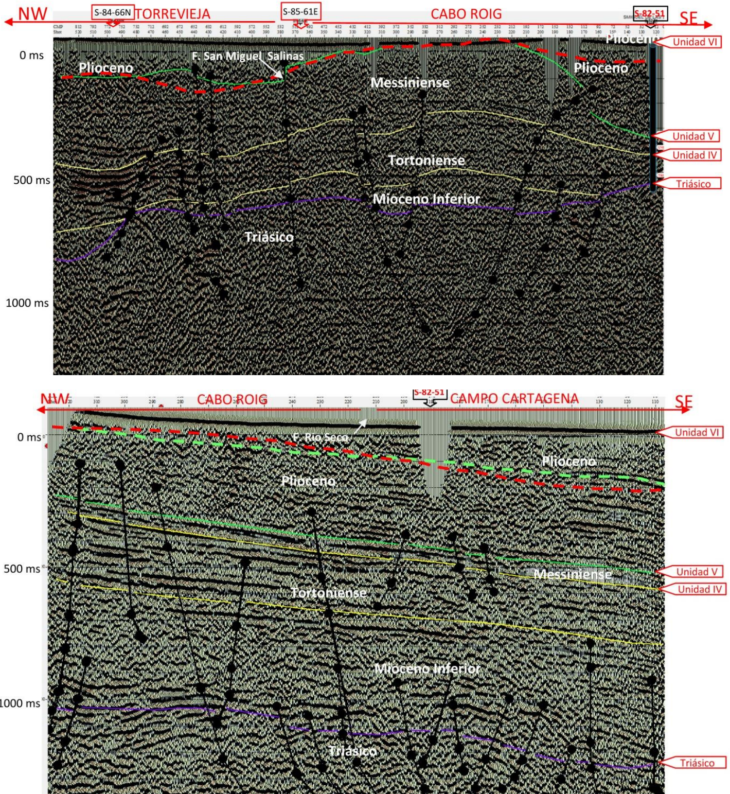
Figura 12. Líneas S-84-66S (arriba, con sondeo de calado) y S-86-90 (abajo). Se indican techos de Unidades. Rojo: muro (independiente) del acuífero Plioceno en modelo 3D Geomodeller.
