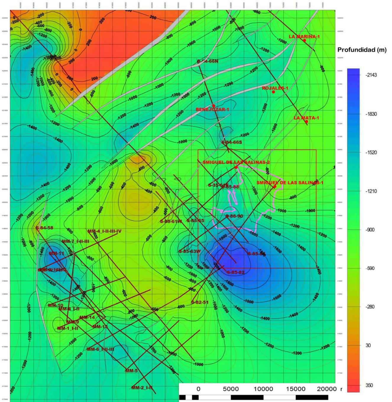
Figura 17. Mapa isobatas Techo Triásico. Se indican las líneas sísmicas usadas en su interpretación. La extensión corresponde al recuadro rojo de la figura 16. Explicación en texto.
