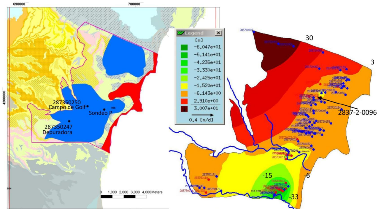
Figura 8. A la izquierda: mapa de índice de salinidad según norma Riverside (US Salinity Laboratory, 1954). Rojo indica salinidad extrema (intrusión marina); azul claro, salinidad media (agua apta para uso agrícola y doméstico). Modificada del informe %Actualización de la geometría del acuífero de Cabo Roig y caracterización litoestratigráfica de los sondeos realizados en la zona sur del acuífero. (DPA-IGME, 2007a)±
