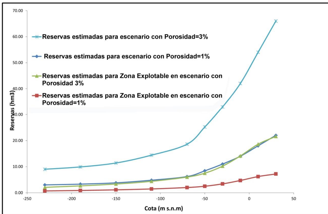
Figura 23. Curvas de reservas del acuífero Plioceno de Cabo Roig obtenidas a partir del modelo geológico 3D del acuífero.
